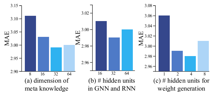
Fig. 11. Evaluation of parameter settings on METR-LA.
