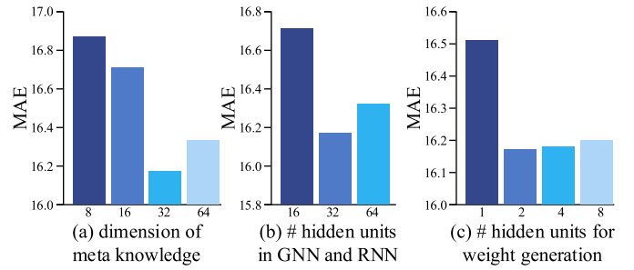
Fig. 10. Evaluation of parameter settings on TAXI-BJ.
