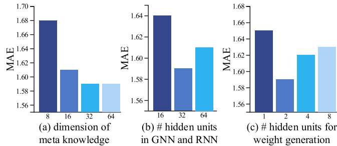
Fig. 12. Evaluation of parameter settings on PEMS-BAY.
